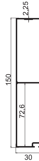
P-101 30x150 Kutu 1,711 kg/m
