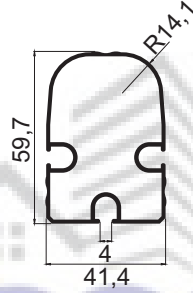
P-104 İnce Korniş 0,937 kg/m
