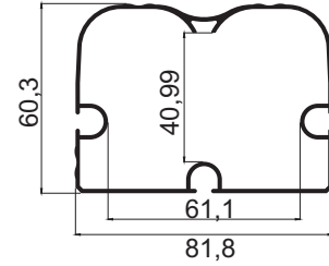
P-103 Kalın Korniş 1,280 kg/m
