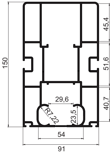
P-102 Orta Seri Ray 5,217 kg/m
