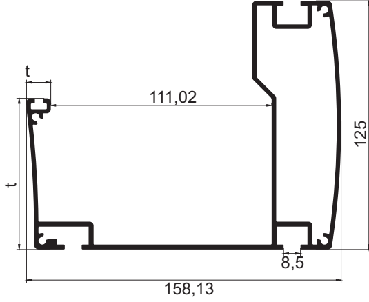
P-106 Orta Seri Oluk 3,916 kg/m
