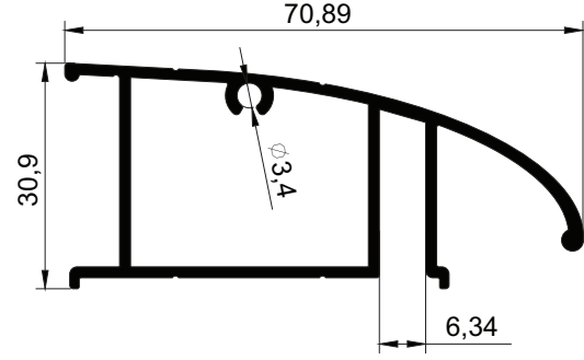
RK-503 KÜPEŞTE 0.806 kg/m
