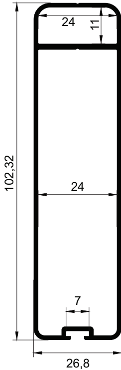
RK-504 AĞIRLIK 1,08 kg/m
